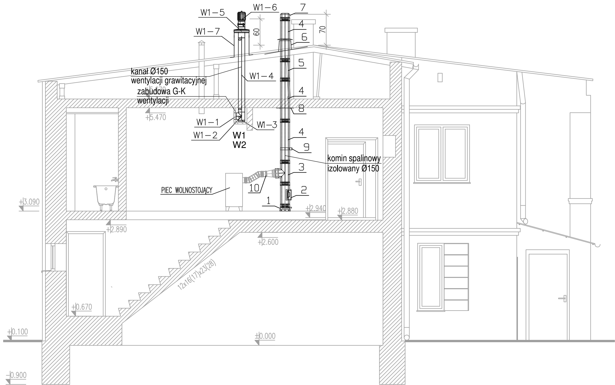
PRZEKRÓJ A-A
